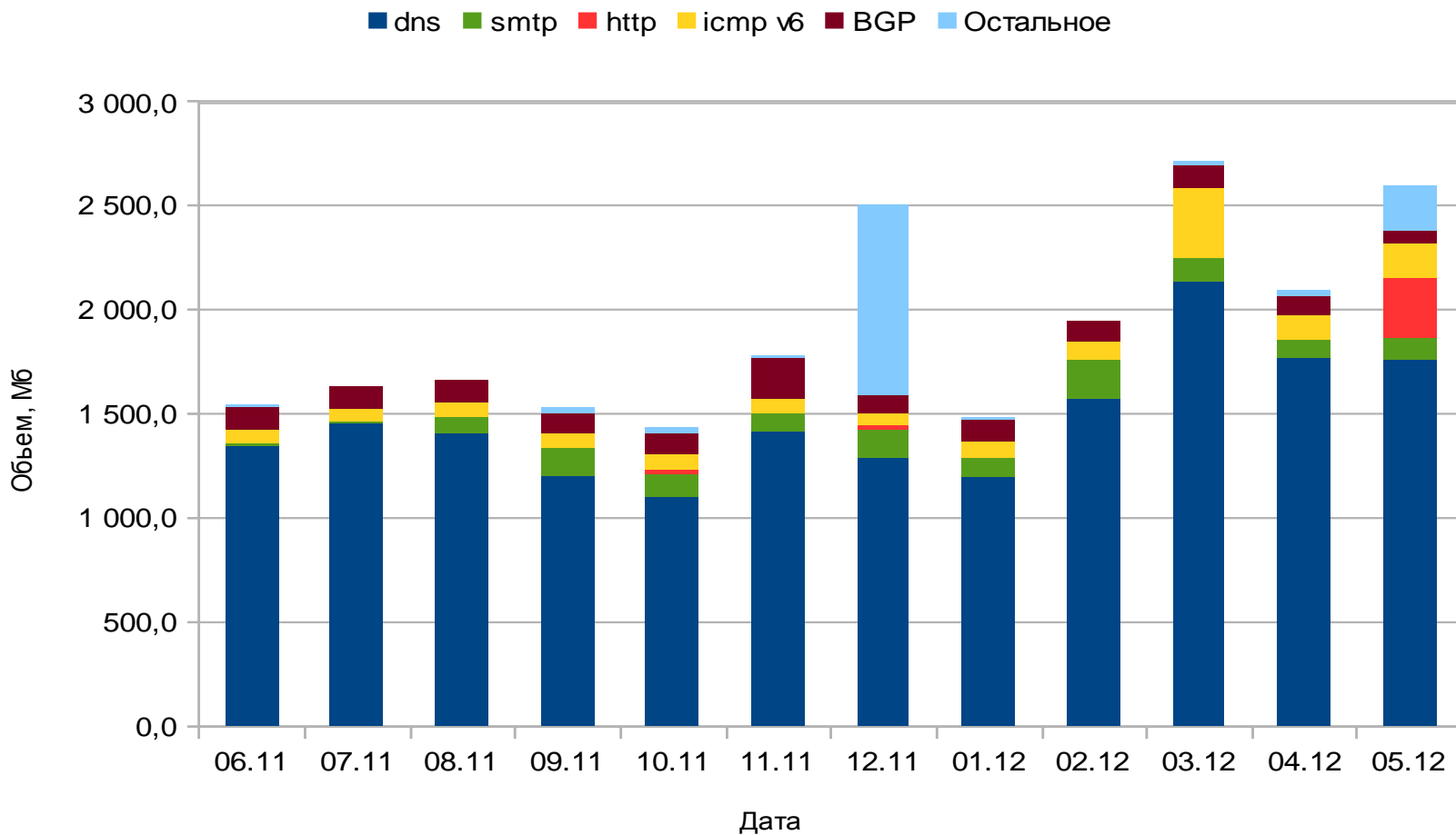
Структура входящего IPv6-трафика
